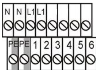
Aansluiting Stroomtoevoer
